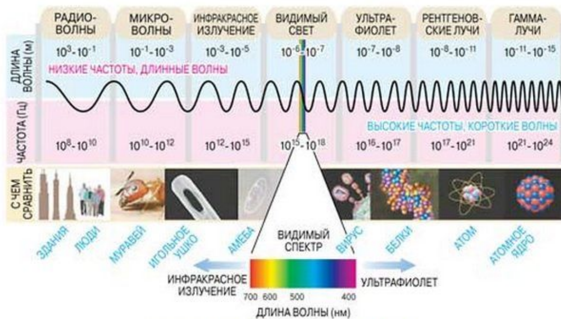
Шкала электромагнитного излучения
